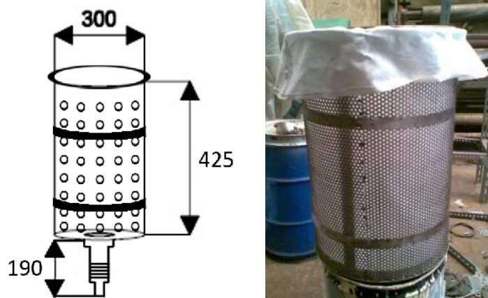
Gambar 8. Tabung pemutar
