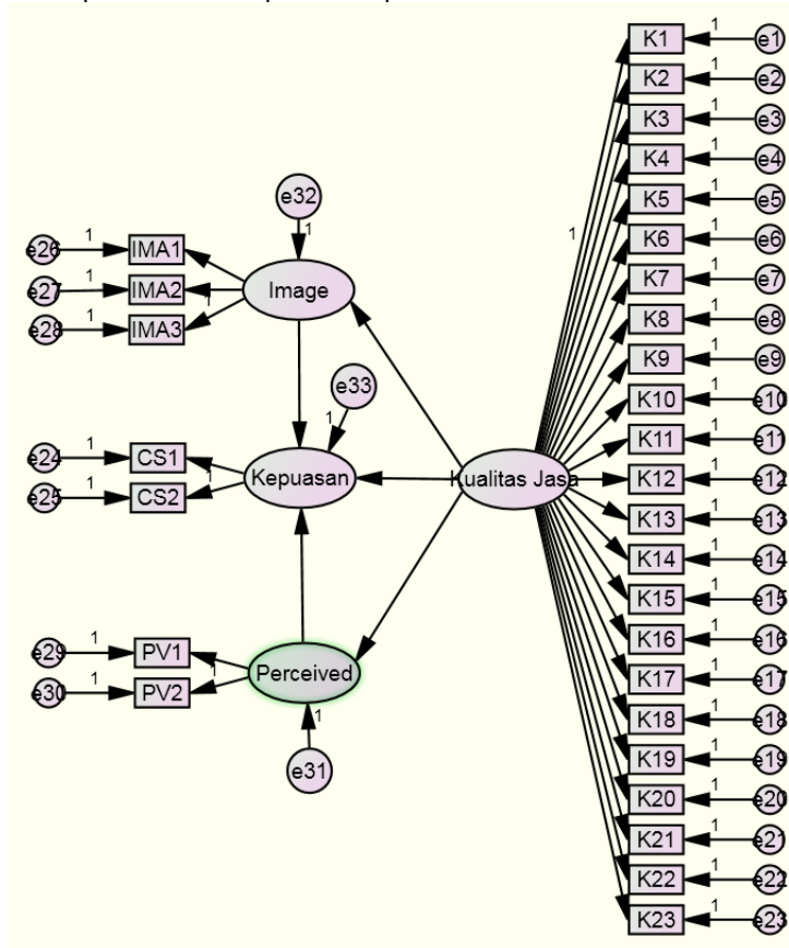
Gambar 2. Model Struktural Kepuasan Konsumen
