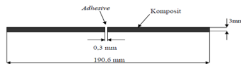
Gambar 3. Sambungan lurus ASTM 5868-95
