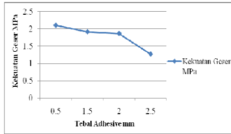
Gambar 3. Sambungan Tumpang
