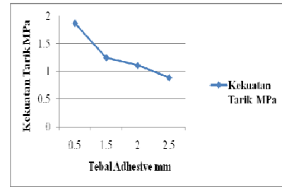
Gambar 4. Sambungan lurus
