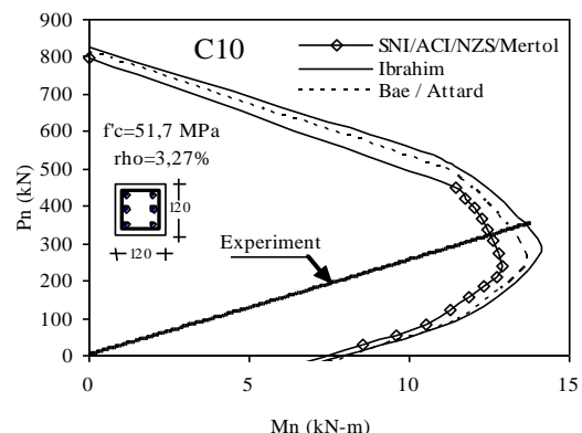
(d) Column C10; \rho=3.27\% , e/h=0.42
