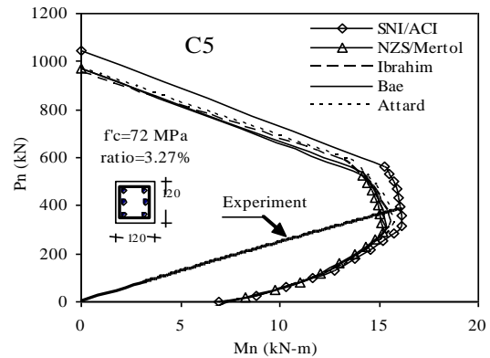
(d) Column C5; \rho=3.27\% , e/h=0.42
