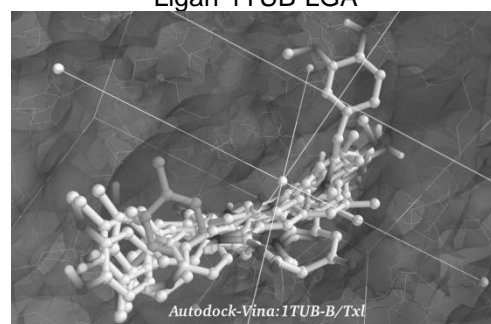
Ligan-1TUB-Vina
