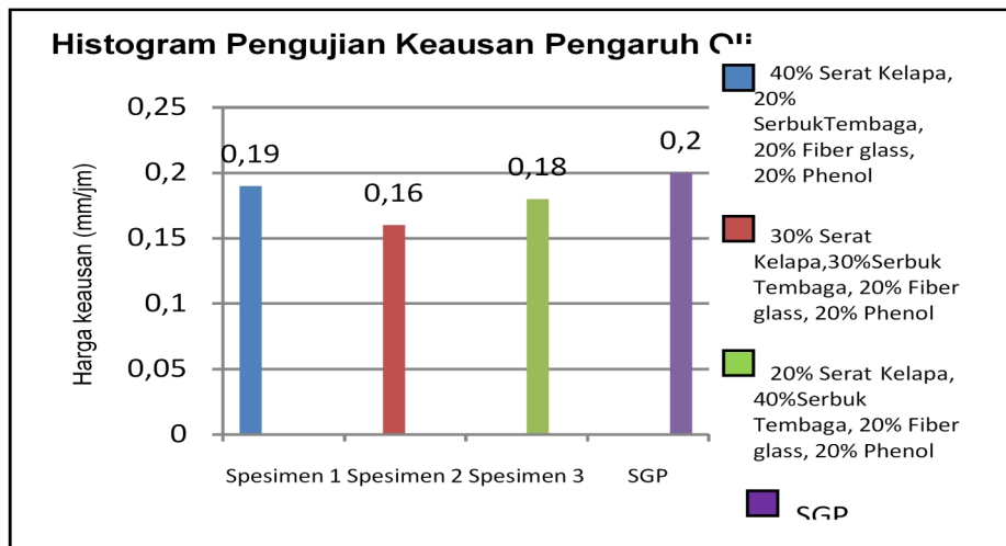
Gambar 2. Histogram Hasil uji Keausan Pengaruh Oli
