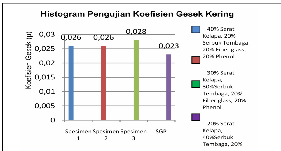
Gambar 3. Histogram Hasil koefisien gesek kering
