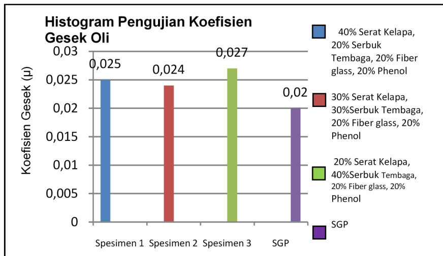
Gambar 4. Histogram Hasil koefisien gesek oli
