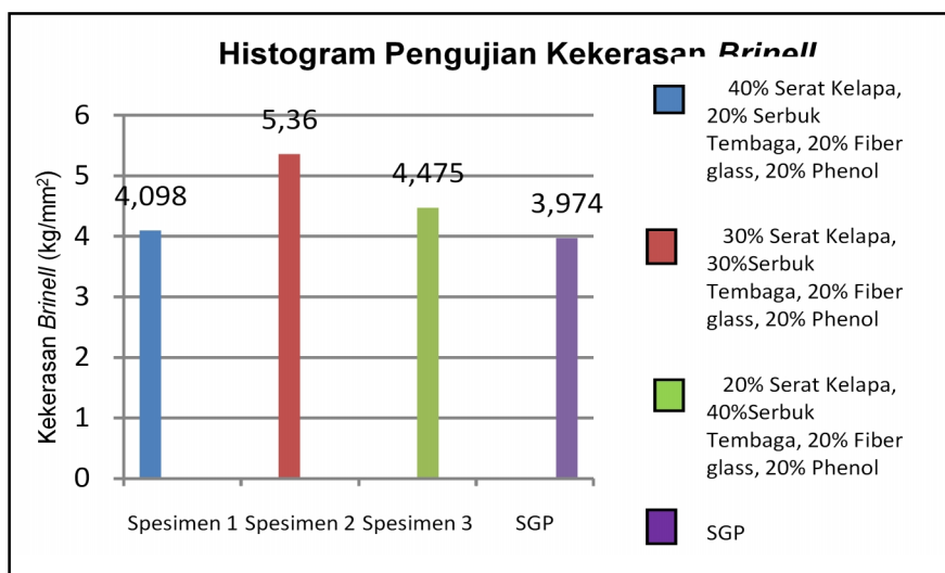
Gambar 5. Histogram Hasil uji kekerasan
