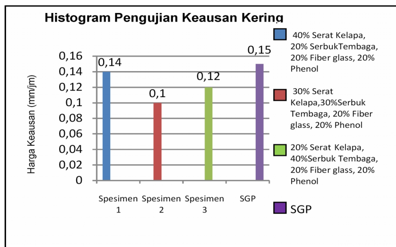
Gambar 1. Histogram Hasil Pengujian Keausan kering
