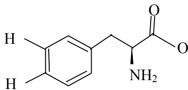
Gambar 2. Struktur molekul L-Dopa
