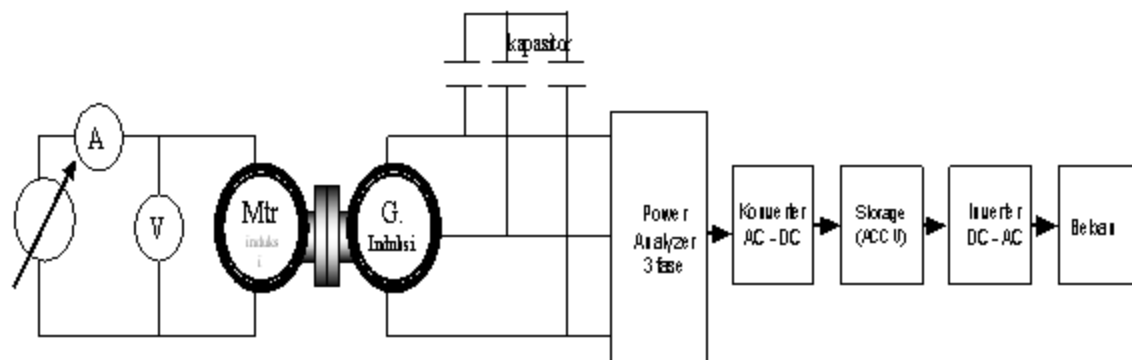
Gambar 3 Rangkaian uji generator berbeban dengan storage
