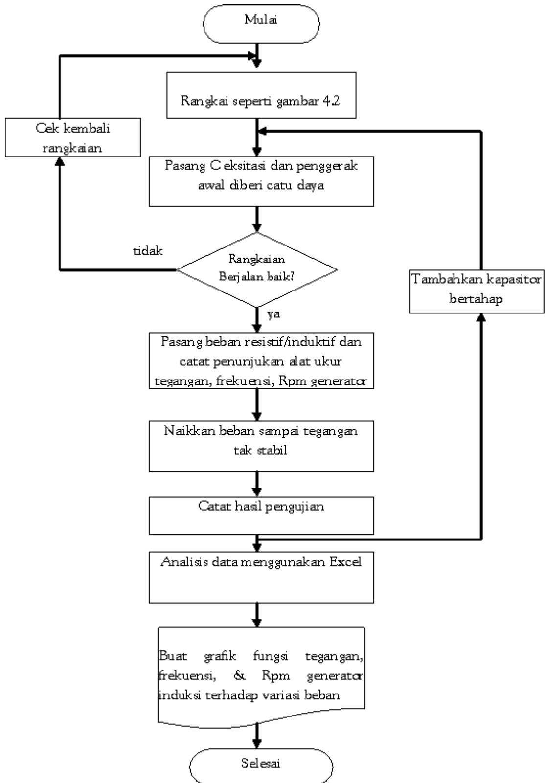
Gambar 5 Diagram Alir Generator Induksi Berbeban Tanpa Storage
