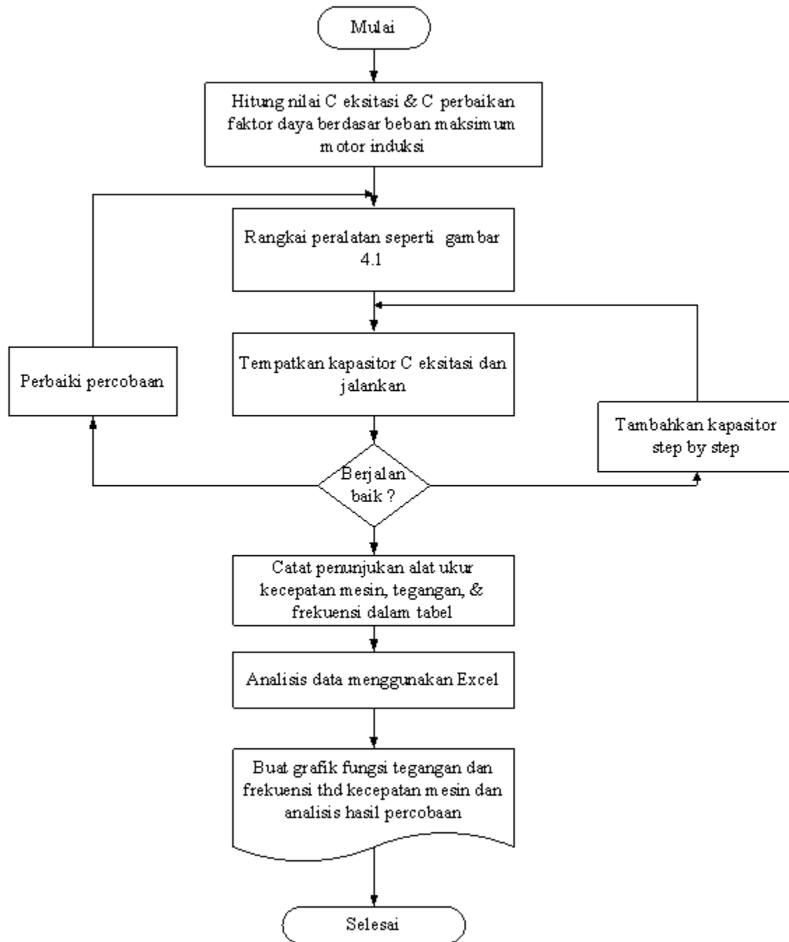
Gambar 4 Diagram Alir Uji Generator Induksi Tanpa Beban
