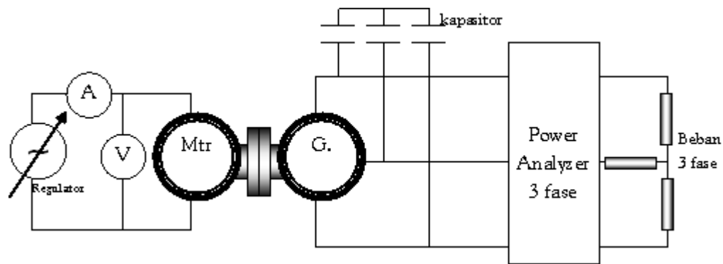
Gambar 2 Rangkaian Uji Generator Berbeban Tanpa Storage
