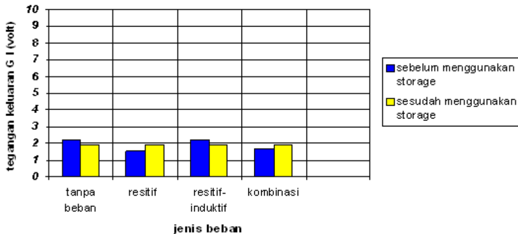
Gambar 7. Perbandingan Tegangan Keluaran Generator Induksi Tanpa dan Dengan Menggunakan Storage .
