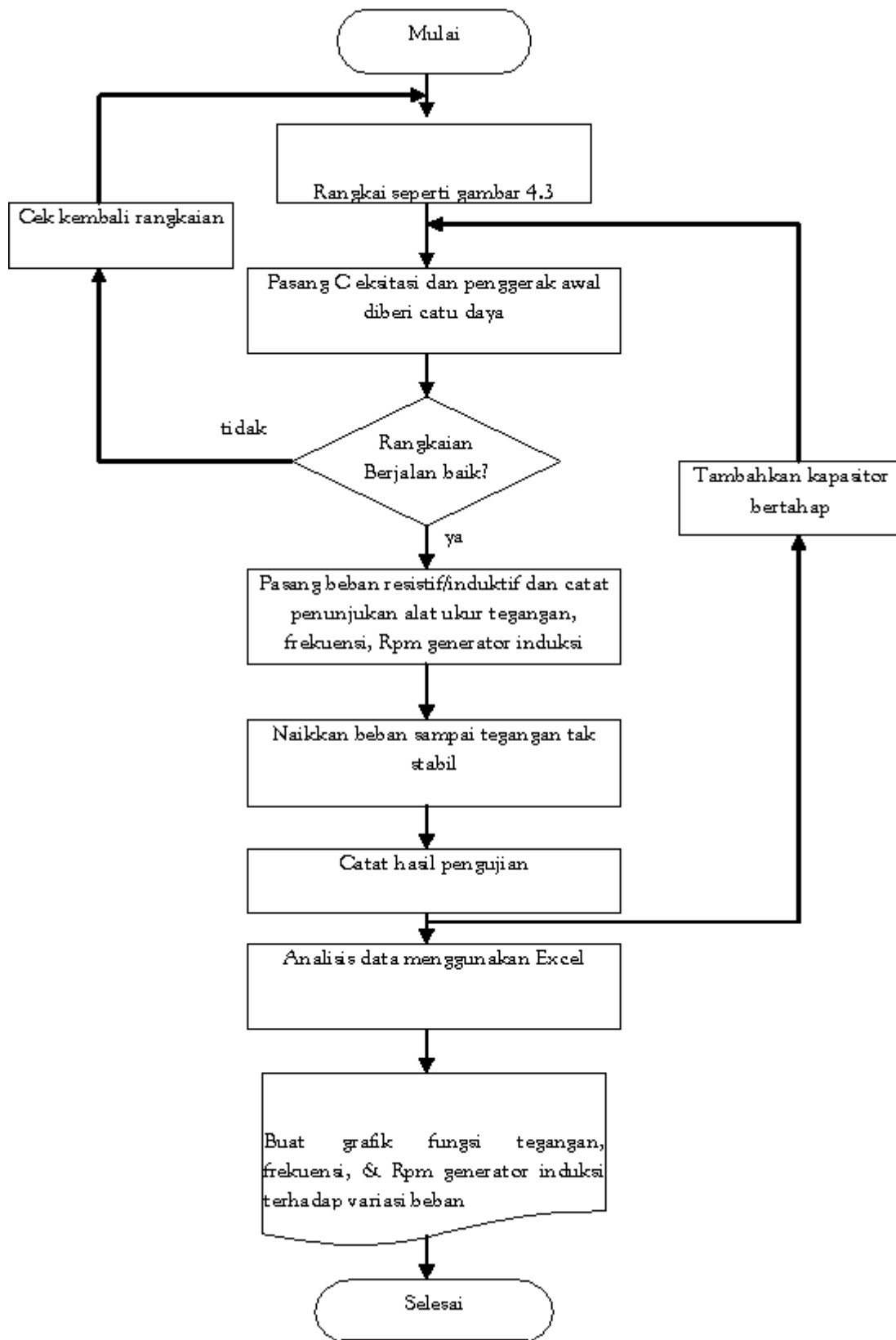
Gambar 6. Diagram Alir Generator Induksi Berbeban Dengan Storage
