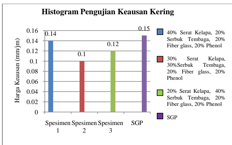
Gambar 2. Histogram hasil pengujian keausan kering
