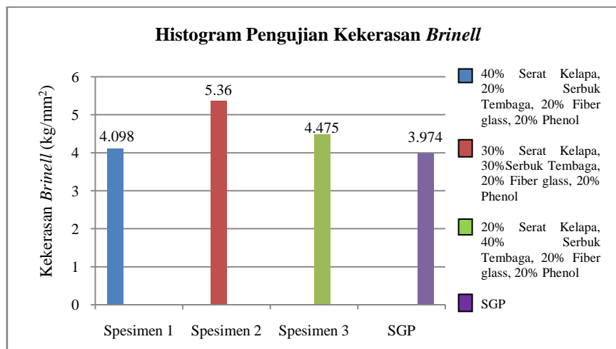
Gambar 6. Histogram hasil uji kekerasan
