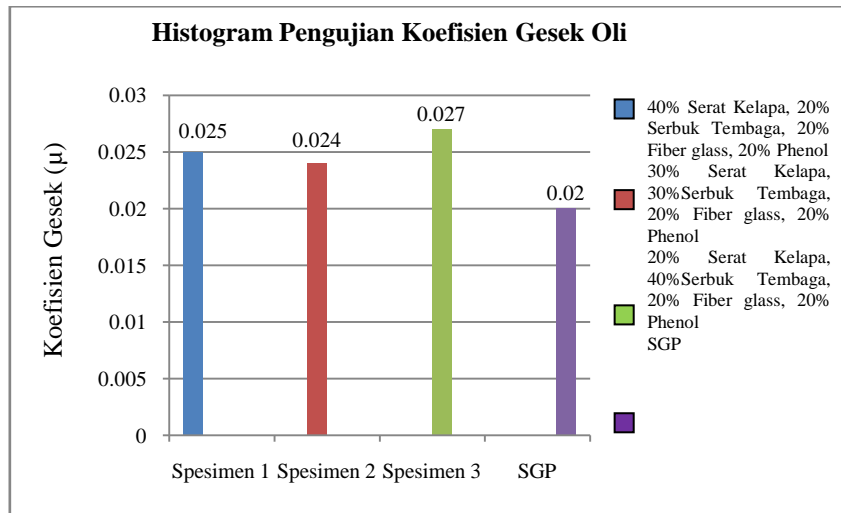
Gambar 5. Histogram Hasil koefisien gesek oli
