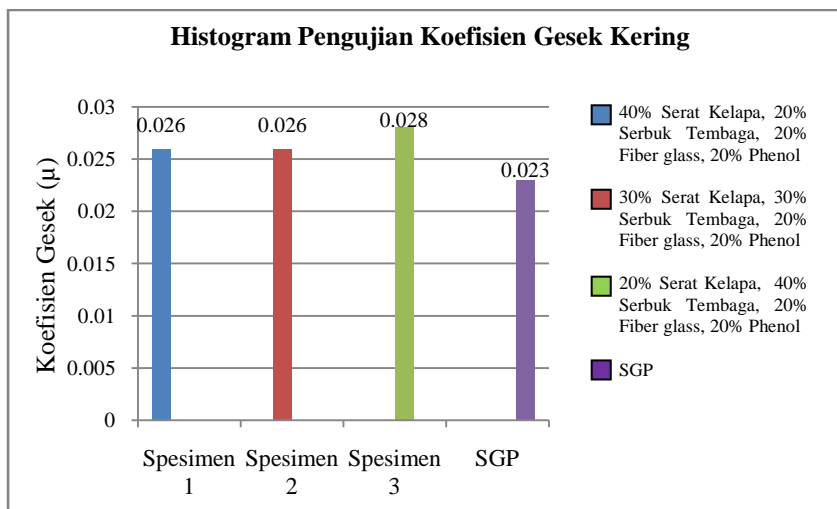
Gambar 4. Histogram hasil koefisien gesek kering
