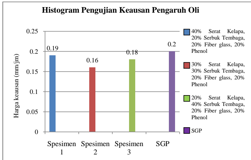
Gambar 3. Histogram hasil uji keausan pengaruh oli
