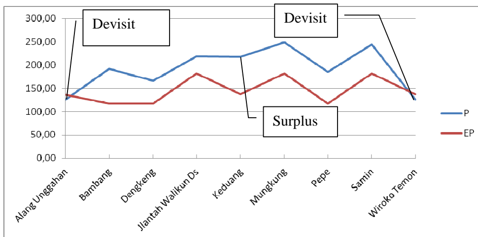
Gambar 2. Grafik Neraca air Umum Wilayah DAS Bengawan Solo Hulu
